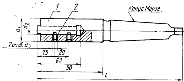
1—оправка; 2—винт по ГОСТ 1477—75
